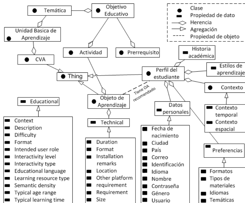
FIGURA 3. Modelo ontológico propuesto.
