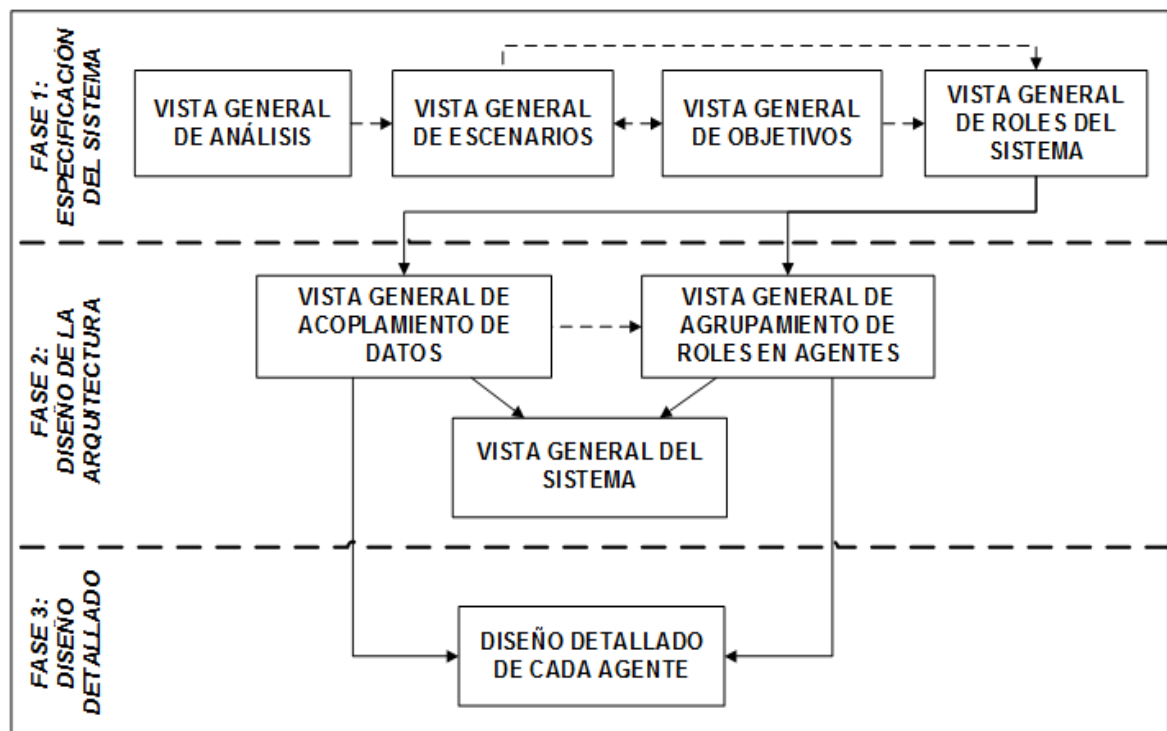
FIGURA 1. Fases de la metodología Prometheus, traducido y adaptado de [22].
