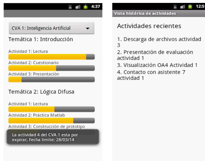
FIGURA 5. Servicios de awareness (Grafo de avance y vista histórica de actividades).
