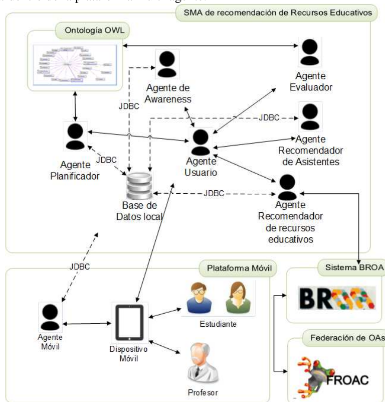
FIGURA 2. Vista general de la arquitectura del sistema utilizando la metodología Prometheus.
